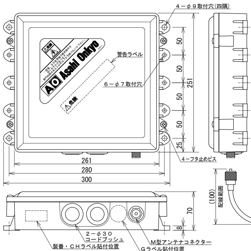
RX-51016G 外形図： ◎RX-61000G、71000G の場合は巻末参照
