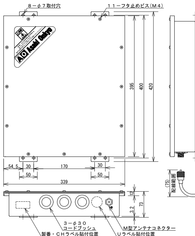
RX-71032U 外形図：
